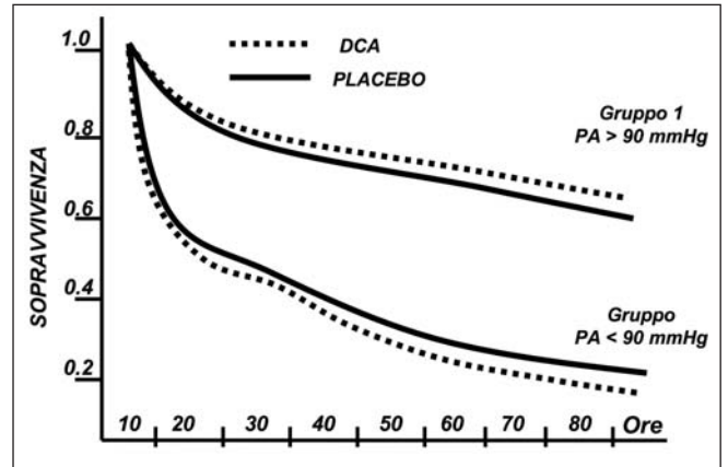
Fig. 5 - Rappresentazione grafica dei dati dello studio di Stacpoolle sull'effetto del dicloroacetato (DCA) sulla sopravvivenza nei pazienti con acidosi lattica. Lo studio ha dimostrato che non vi era alcuna differenza nella mortalità nei due gruppi trattati e non trattati. La differenza di mortalità era determinata alla presenza di shock e non dalla correzione dell'acidosi determinata dall'uso del DCA. Modificata da (38).
